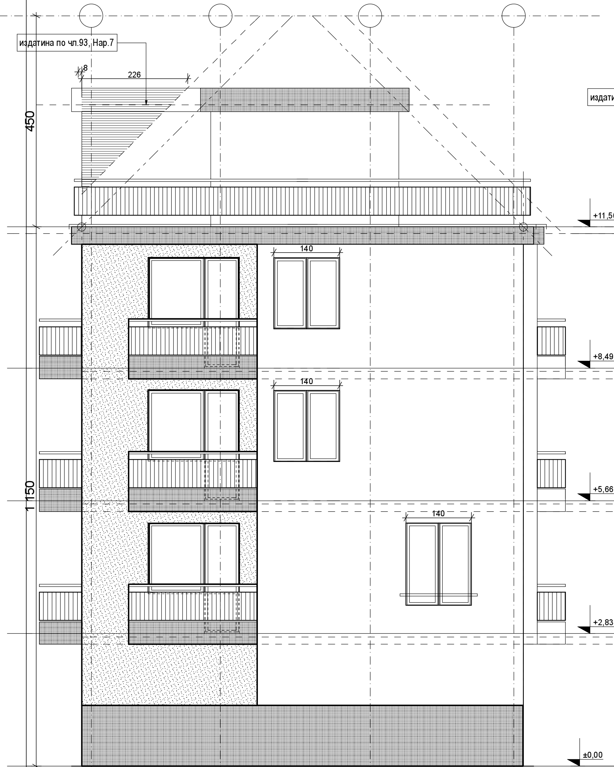
фасада Запад
