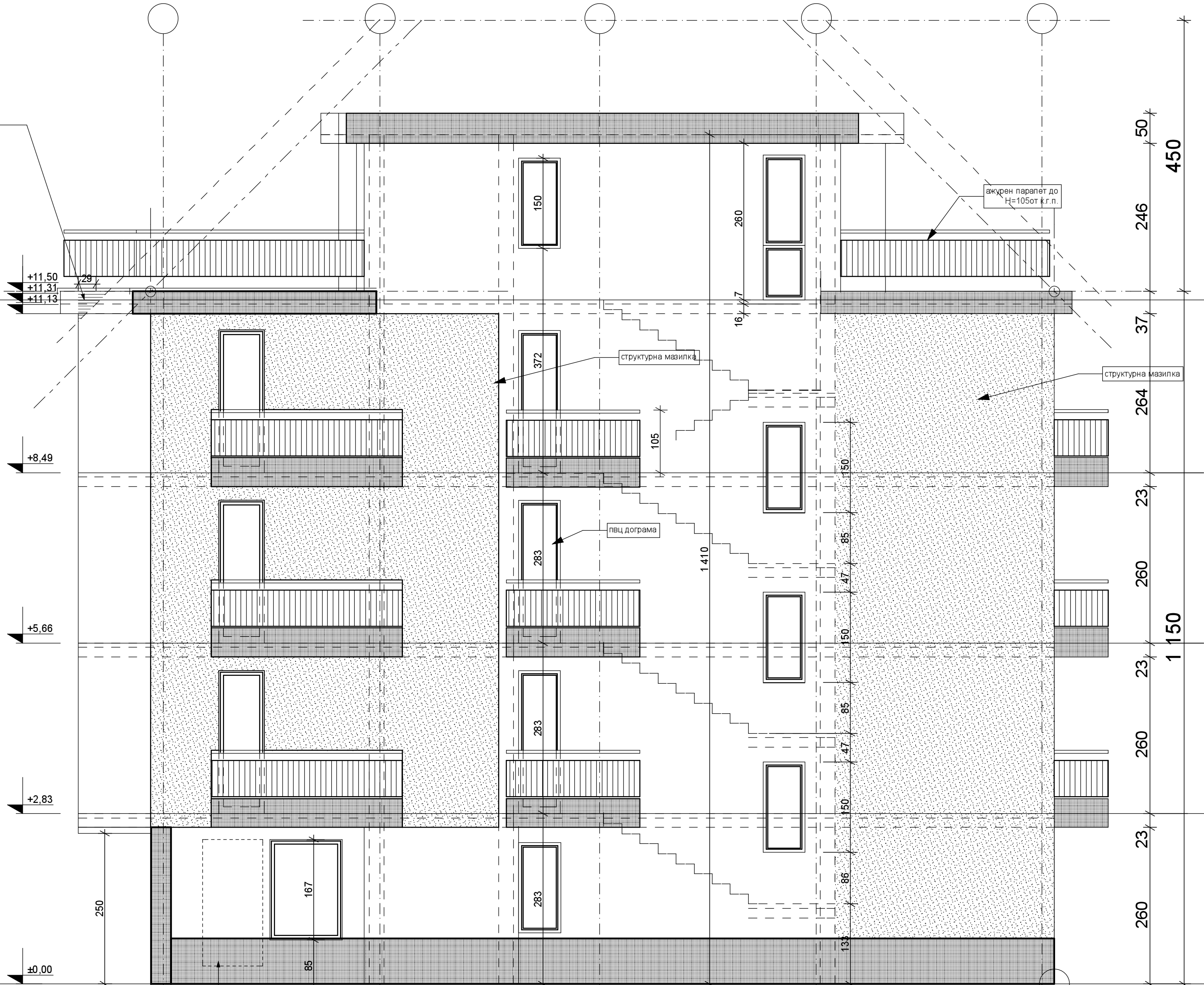
фасада Север
